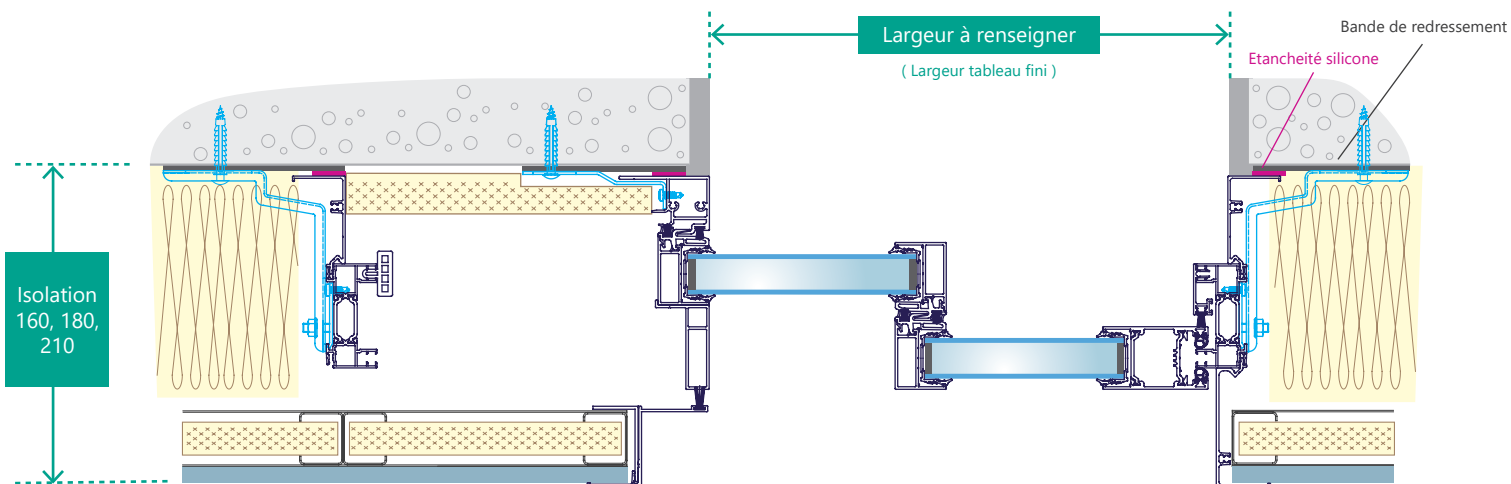
Fig 1. Coupe horizontale
