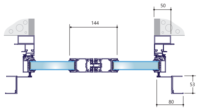
2 vantaux
