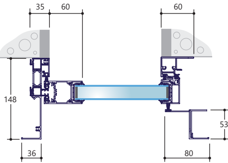
1 vantail
