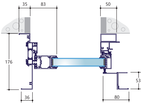
1 vantail
