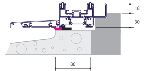
Fig 3. Seuil encastré
