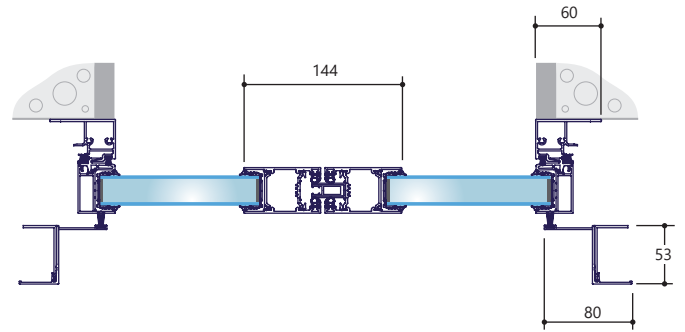
2 vantaux
