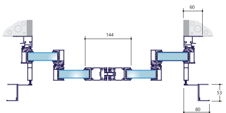
4 vantaux
