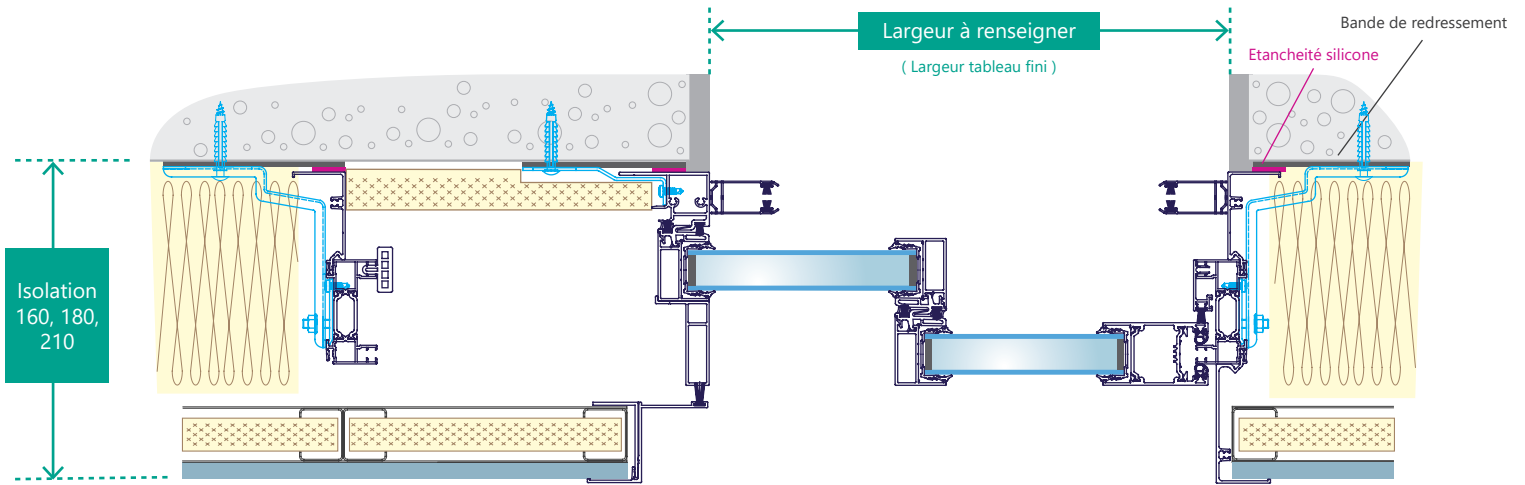
Fig6. Coupe horizontale
