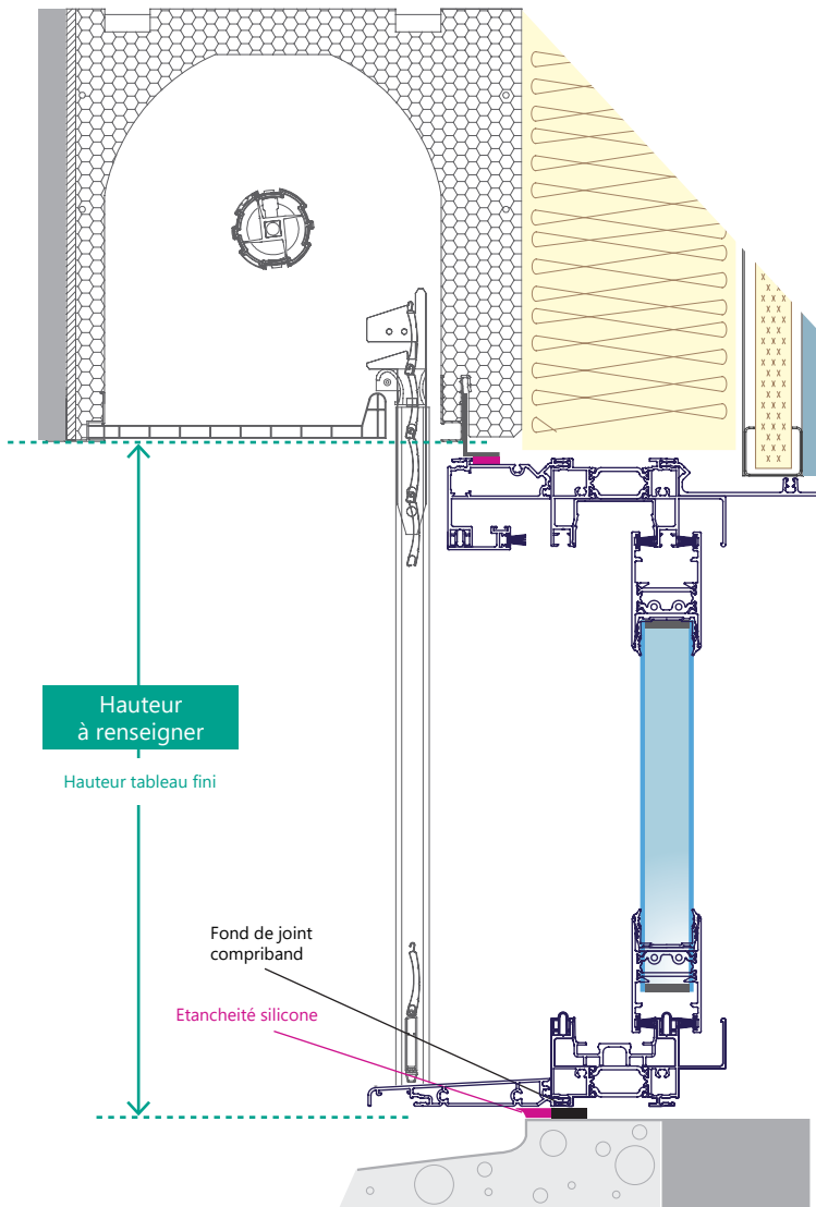
Fig 7. Coupe verticale
