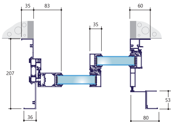
2 vantaux
