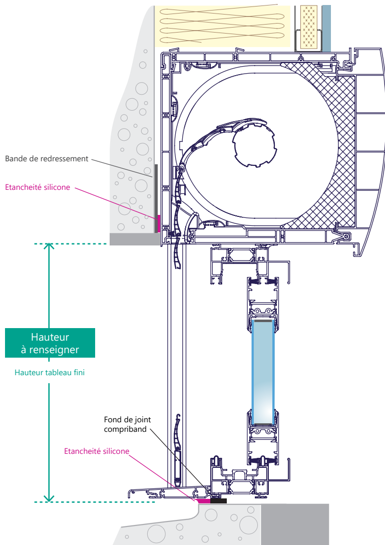
Fig 5. Coupe verticale
